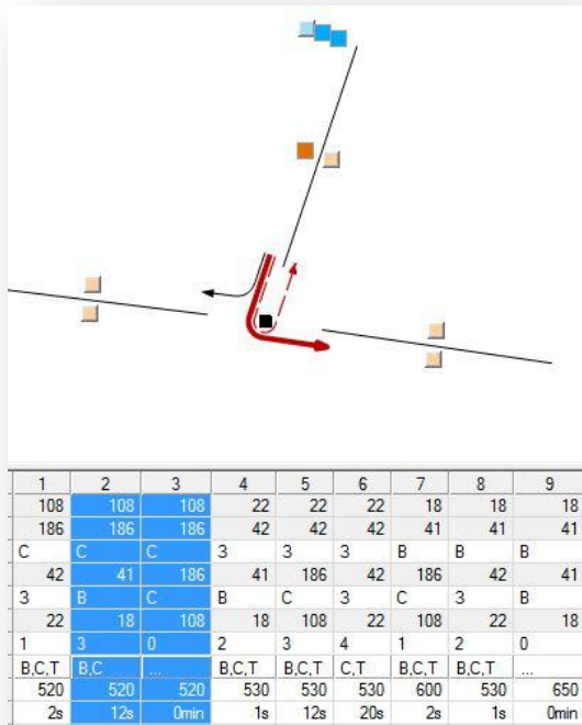
Рисунок 3.1.6 – Атрибуты узла
